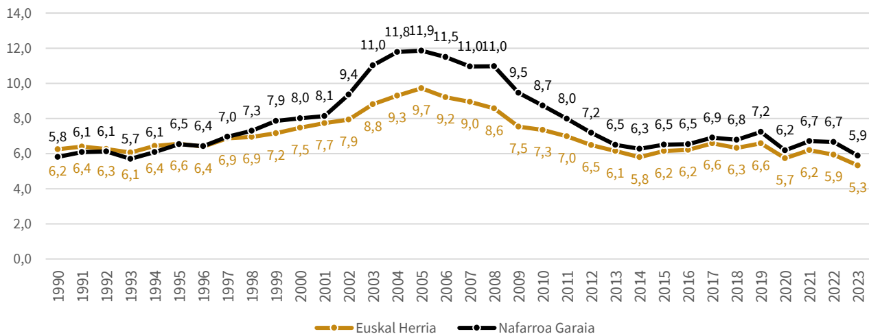
● Berotegi Efektuko Gasen gutzirako isurketen bilakaera (Ktn CO 2 1.000 biztanleko). Nafarroa Garaia eta Euskal Herria 1990-2023 (%)
